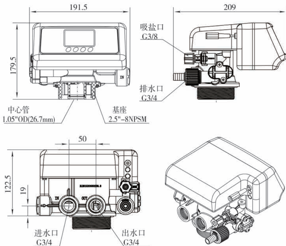
F117A1结构图
